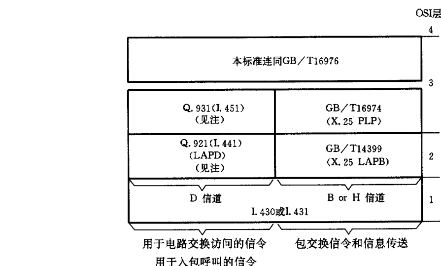
图3 ISDN 中使用 B 信道或 H 信道时在 S 和 T 参考点的协议层
