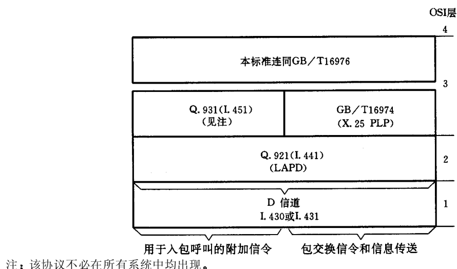
图2 ISDN 中使用 D 信道时在 S 和 T 参考点的协议层
